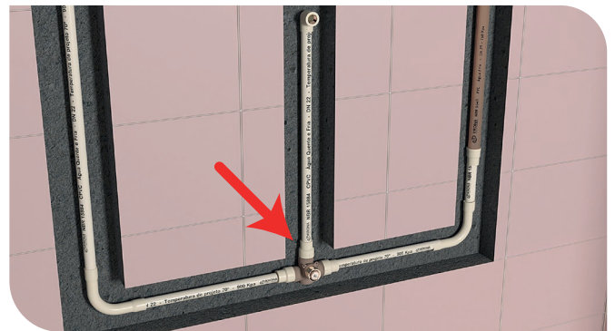
Transição soldável com a Luva de Transição CPVC x PVC.
