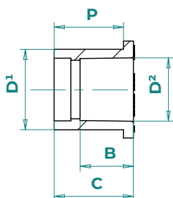
BUCHA DE REDUÇÃO CURTA CPVC ULTRATERM KRONA® DIMENSÕES (mm)
