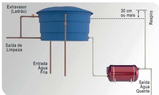
Exemplo de obra horizontal até dois pavimentos: Sistema de aquecimento com aquecedor de acumulação.
