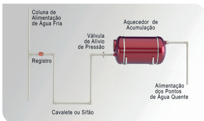
Exemplo de obra vertical prédios: Sistema de aquecimento com aquecedor de acumulação.
