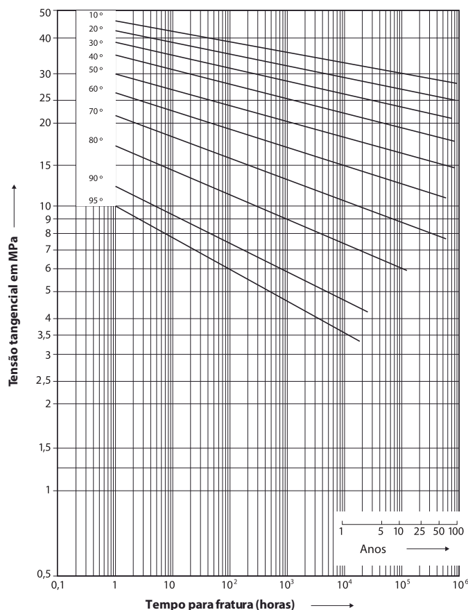
Figura 01 - Curvas de referência para a resistência à pressão hidrostática interna esperada para tubos de CPVC
