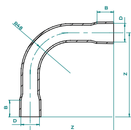
CURVA 90° CPVC ULTRATERM KRONA® DIMENSÕES (mm)
